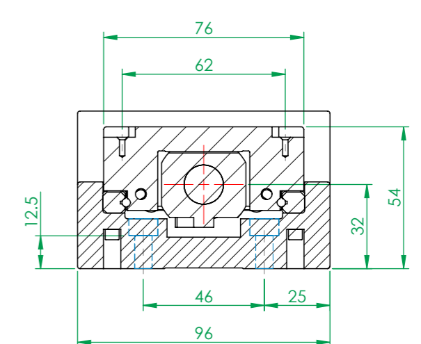
剖面圖 K-K
