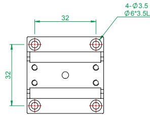
MX(Y)40-S系列 底座安裝孔尺寸
