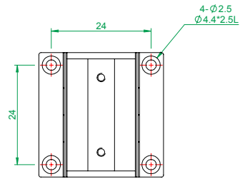
MX(Y)30-S系列 底座安裝孔尺寸
