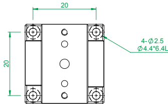
MX(Y)25-S系列 底座安裝孔尺寸
