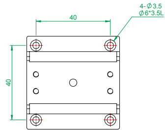
MX(Y)50-S-28系列 底座安裝孔尺寸
